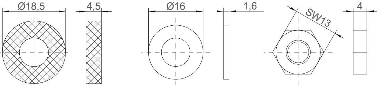
* Einschraubhilfe für FOPPE-Befestigungsbolzen Artikel-Nr.: 140106903
