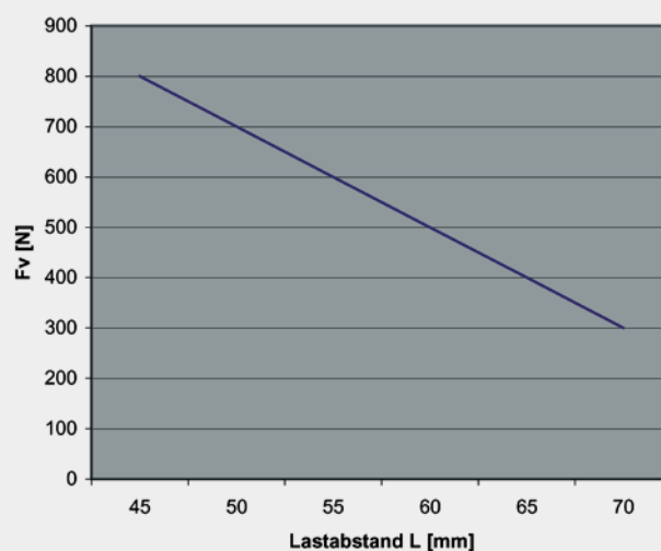
Maximale Vertikalkraft Richtwerte auf Basis System Schüco
