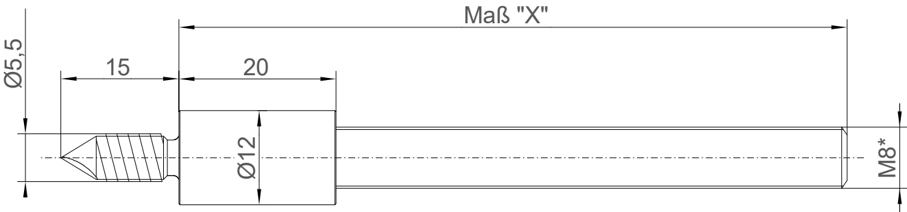
* Einschraubhilfe für FOPPE-Befestigungsbolzen Artikel-Nr.: 140106903
